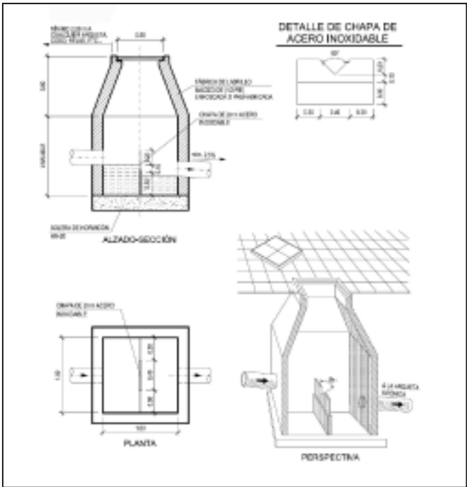
ANEXO NÚM.2 MODELO DE ARQUETA DE TOMA DE MUESTRA
